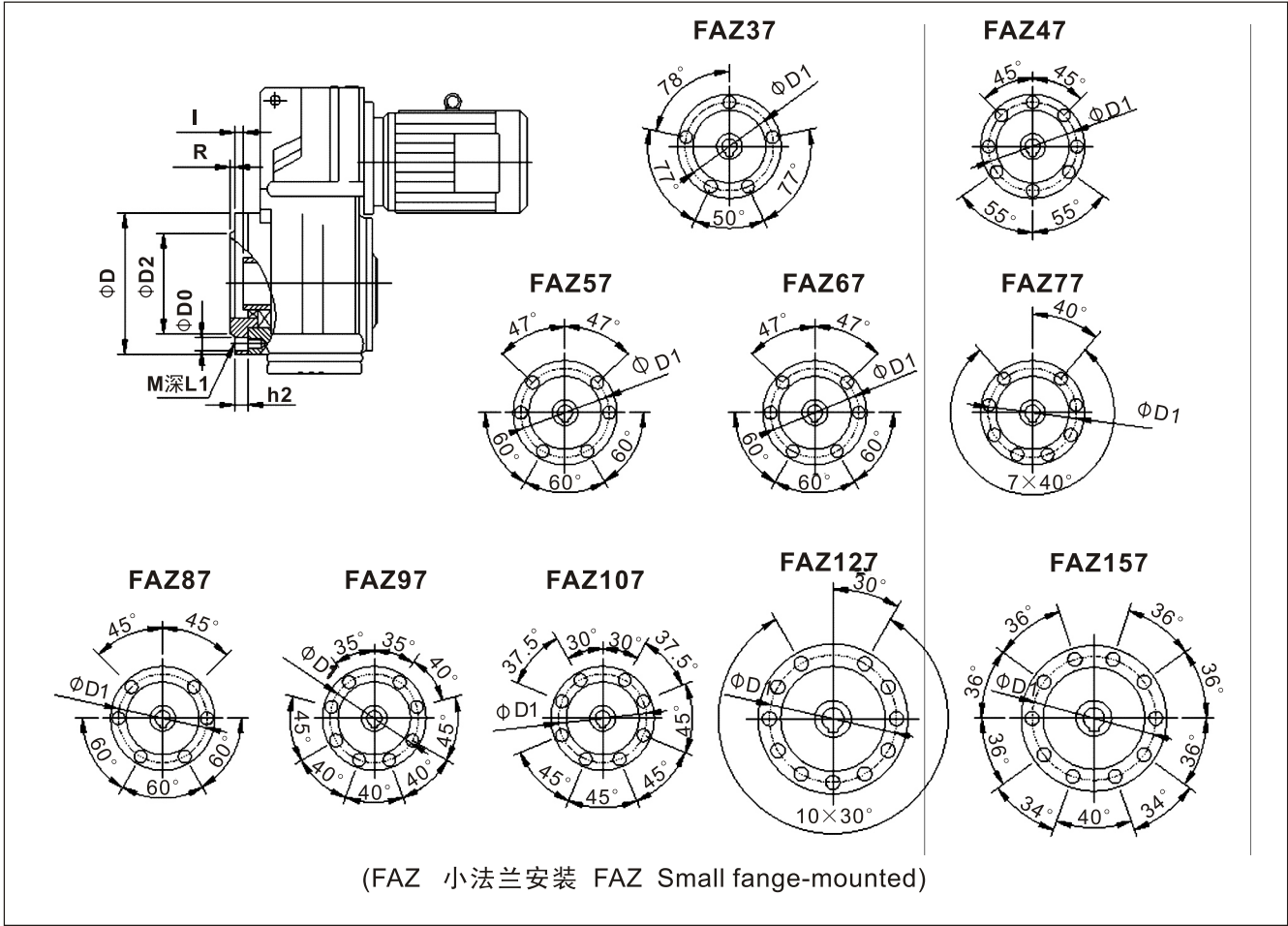
外形安装尺寸:
